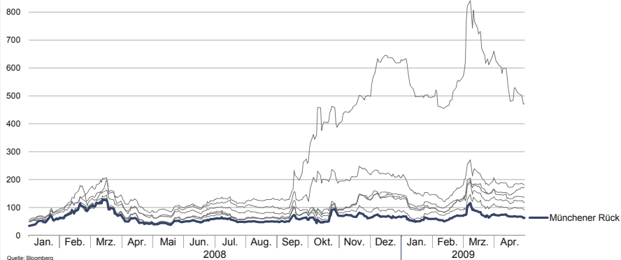
CDS-Zinsaufschläge 1 (1.1.2008–30.4.2009) 2
